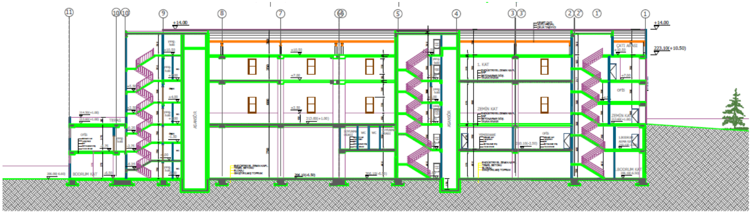
A-A KFSİTİ 1/100
